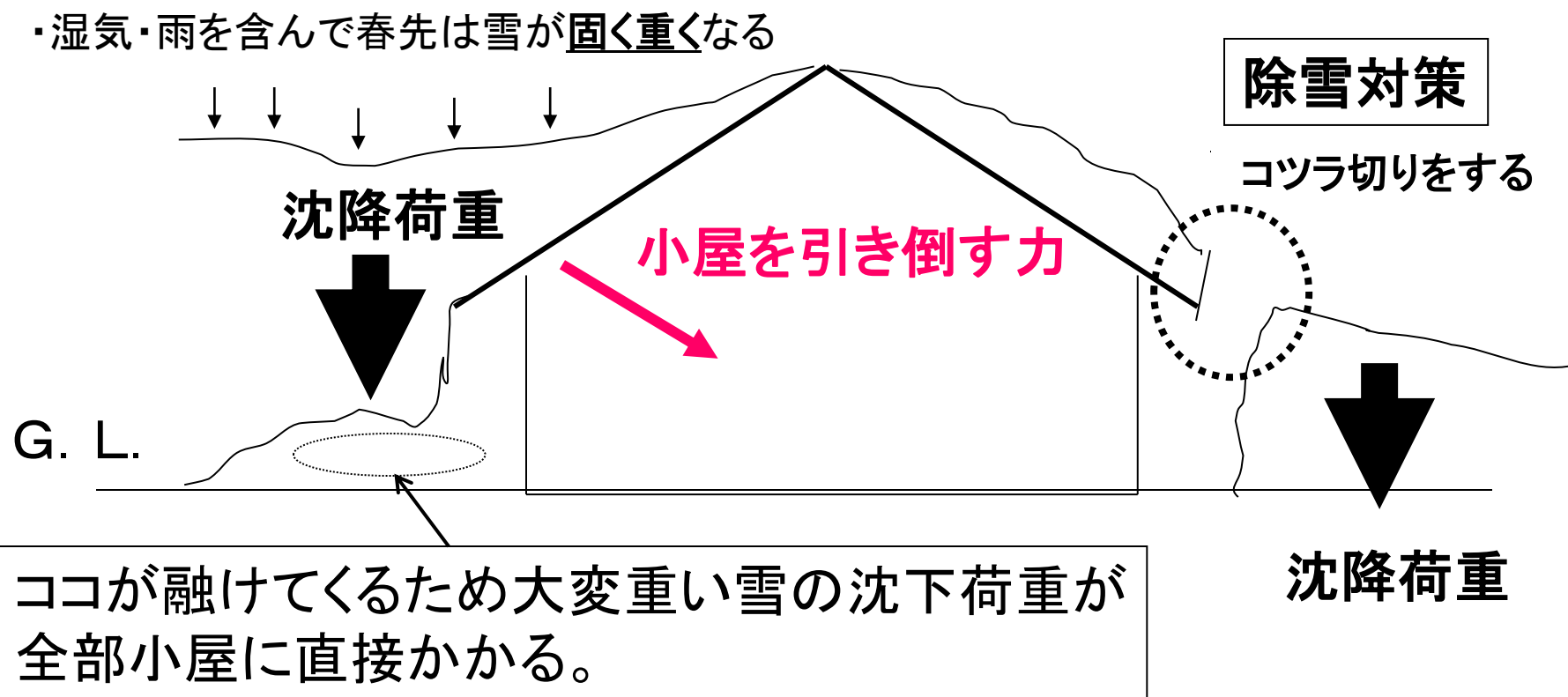
図2 春先の小屋倒壊メカニズムとコツラ切りの重要性
