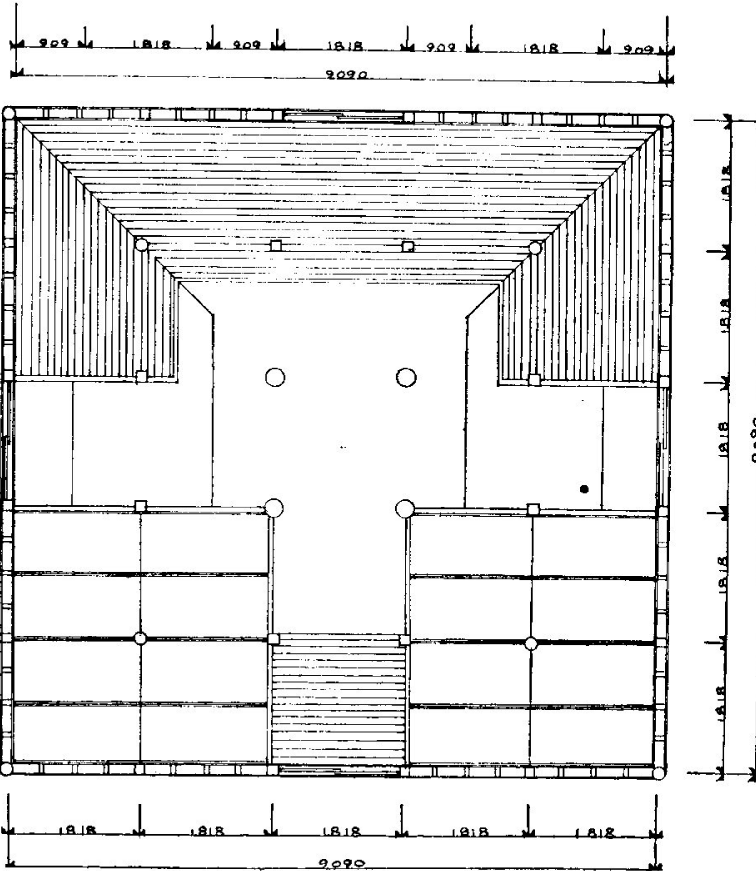
2階平面図
