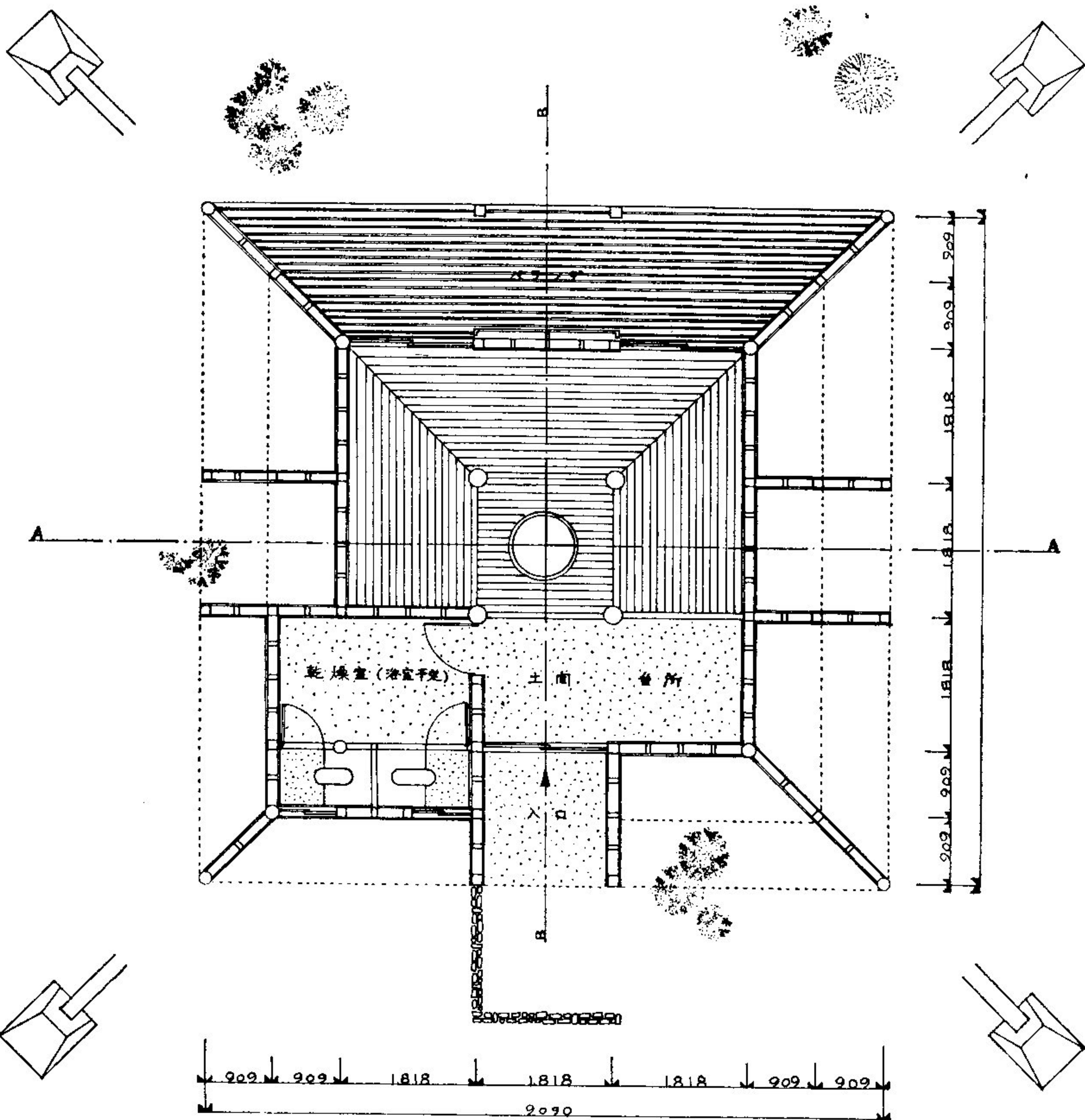
1階平面図
